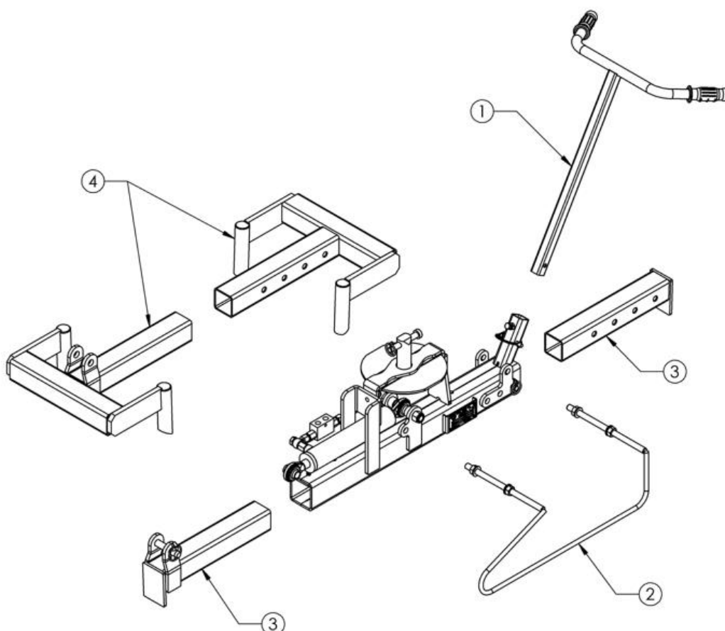
Figuur 1 Boordsteen- grasdalklem met standaard toebehoren
